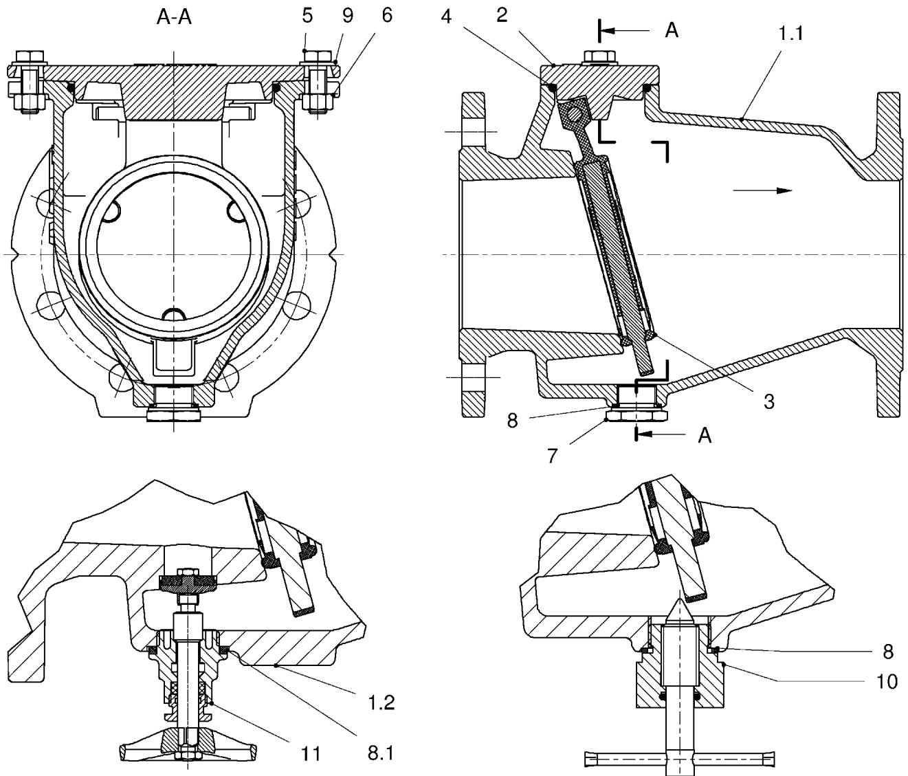
Version: mit Umführung with by-pass valve
